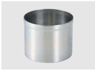
MR-272 ..... ¥1,700 スリムシュガーポット (フタ・レードルなし) 材質/18-8ステンレス 箱サイズ/95×85×H82mm 入数/100 本体サイズ/φ80×H65mm 容量/280ml
